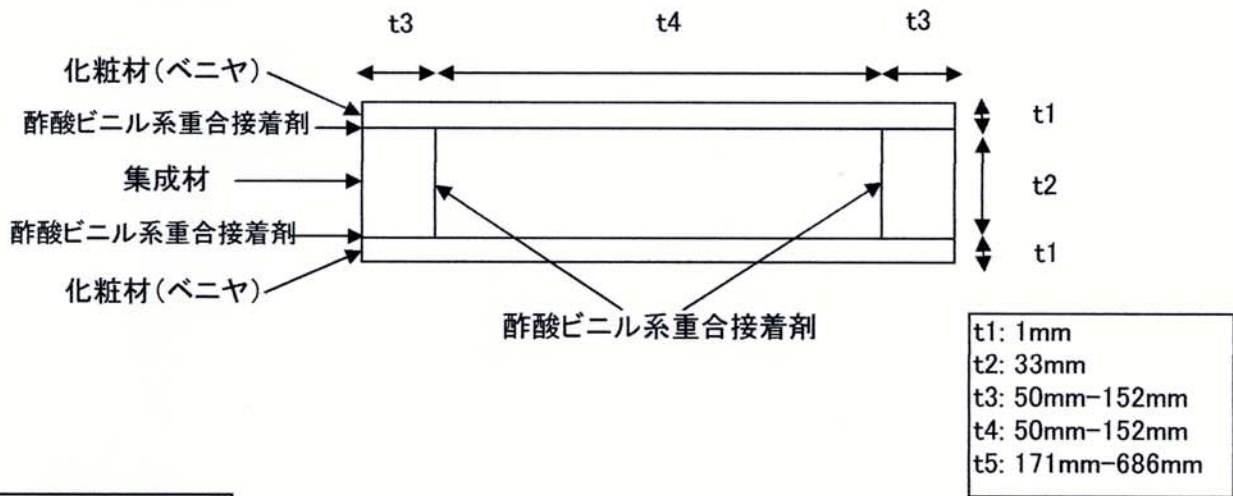
図-3 断面図B
