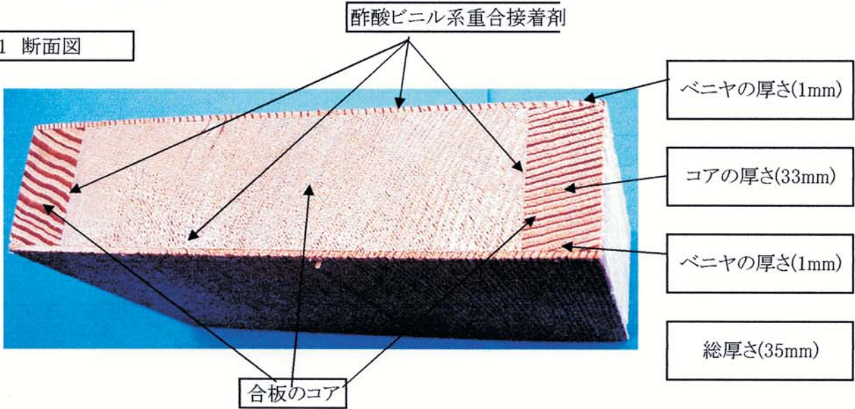
図-2 断面図A
