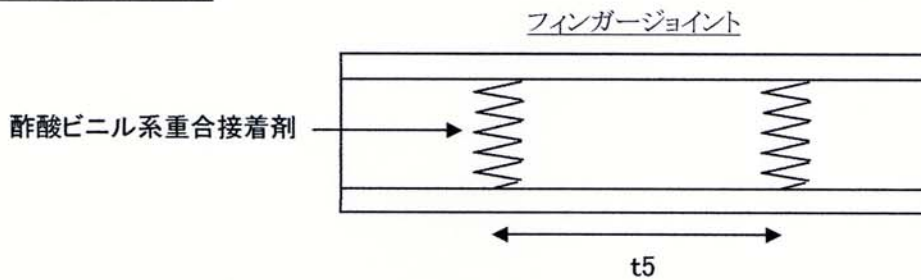
図-3 断面図B
